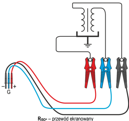
R iso- – przewód ekranowany
