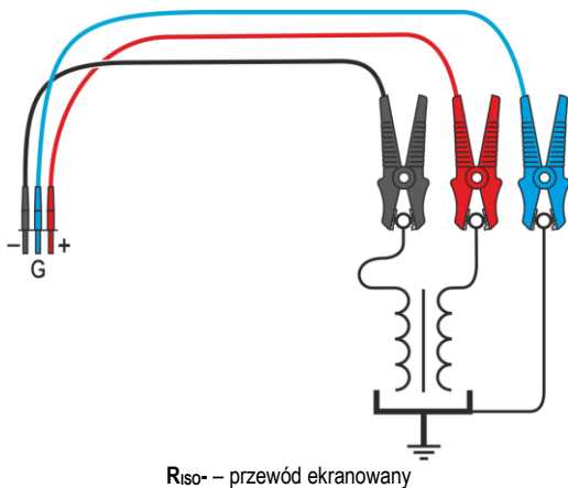
R iso- – przewód ekranowany
